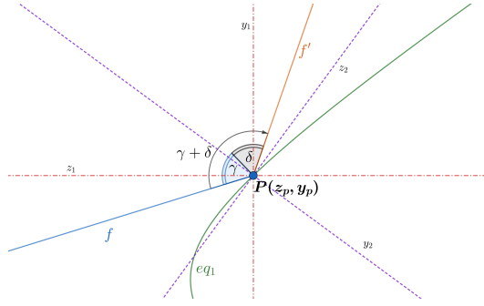
Gambar 4. Transformasi garis f menjadi garis f'
