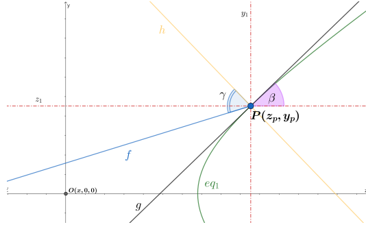
Gambar 3. Translasi sistem koordinat
