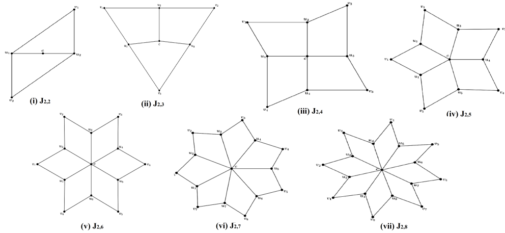
Gambar 1. Graf Jahangir J_{2,m} dengan 2 \leq m \leq 8
